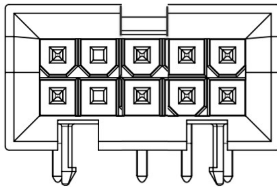
P/N 15-24-9107 10 Ckt
